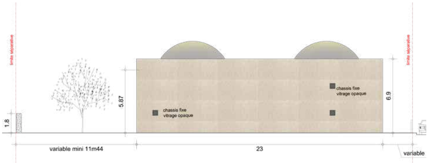
FAÇADE OUEST
