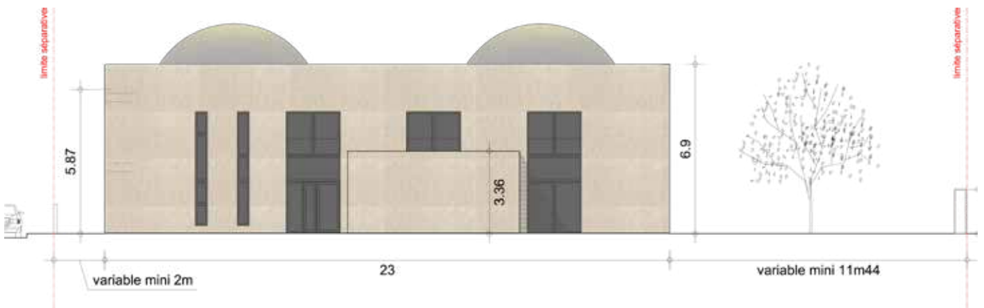
FAÇADE EST
