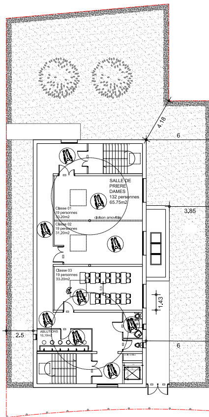
PLAN NIVEAU 01
