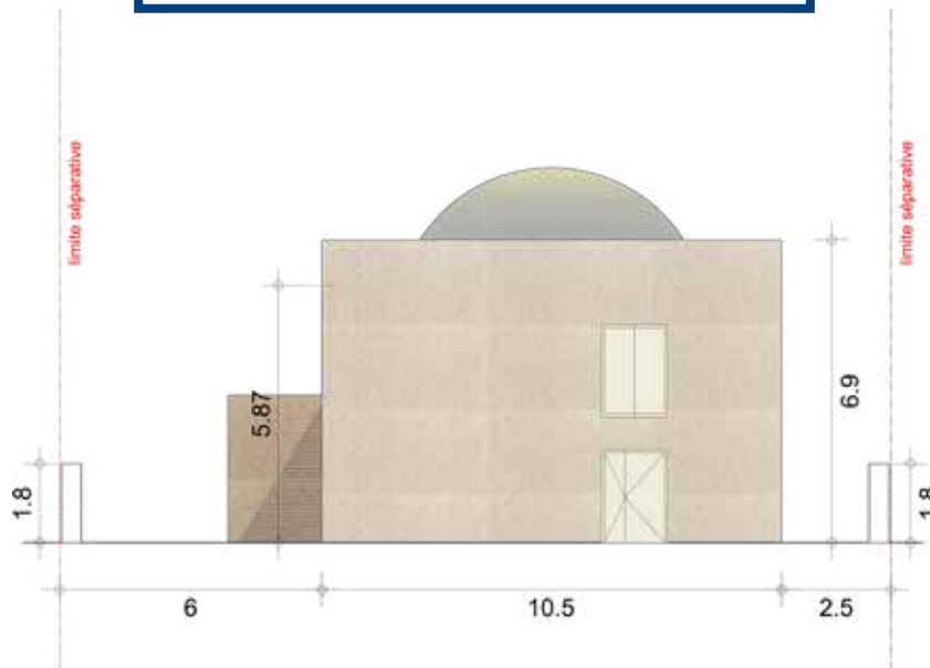
FAÇADE NORD
